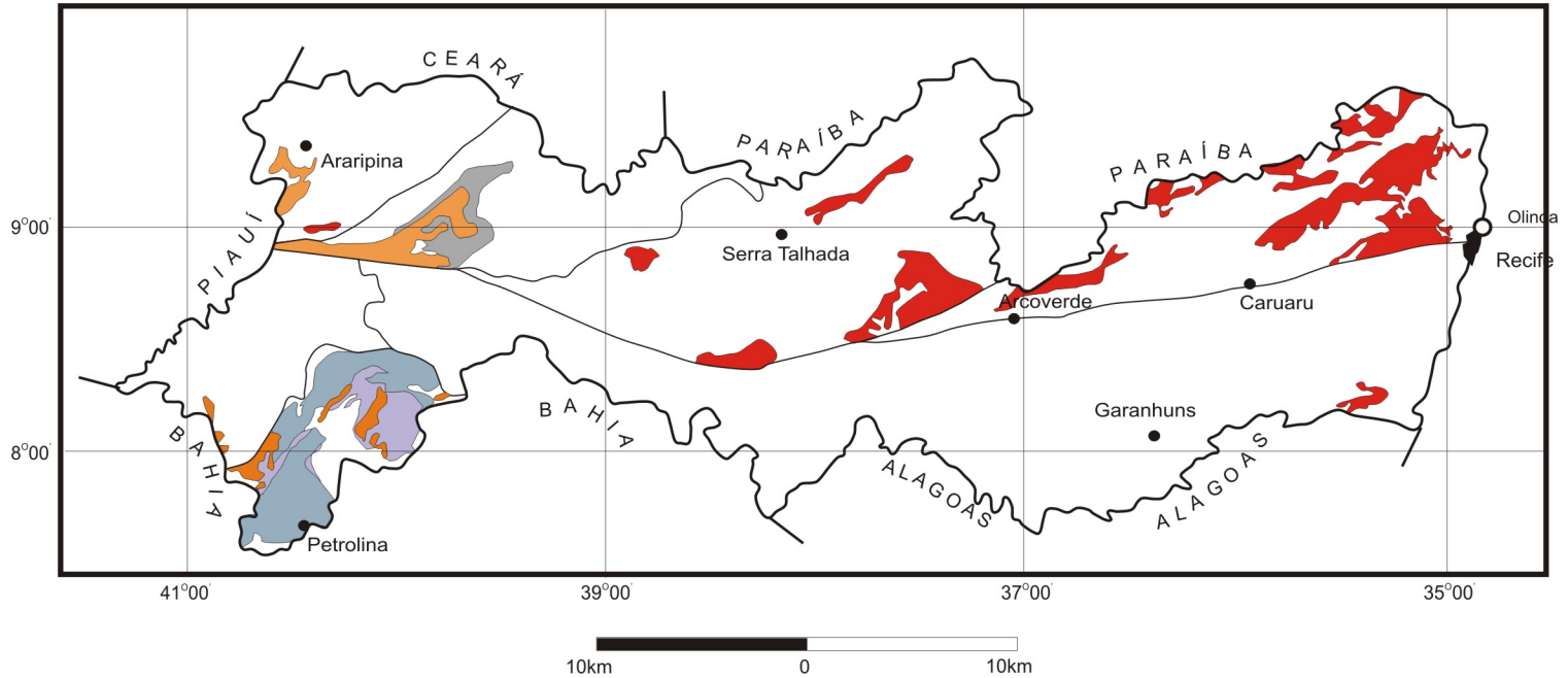
Figura 6 - Arqueano a Paleoproterozóico no Estado de Pernambuco
